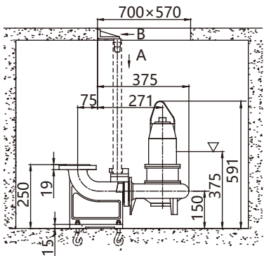
安装尺寸图
