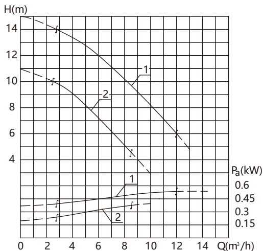
性能曲线图
