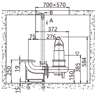
安装尺寸图
